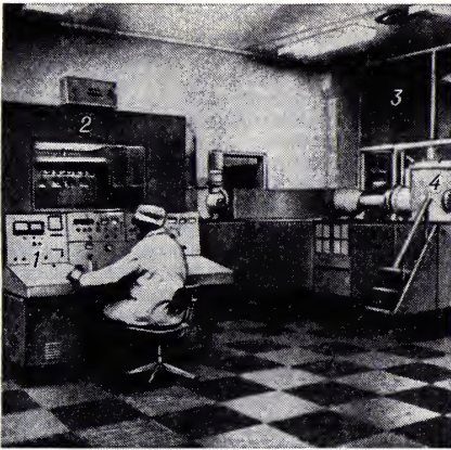
Рис. 1. Универсальная пиннолучевая установка «Везувий-1» (СССР) с энергией ионов до 200 кэв, позволяющая осуществлять ионное легирование полупроводниковых материалов практически любыми примесями: 1 — пульт управления; 2 — источник и ускоритель ионов; 3 — магнитный сепаратор ионов; 4 — камера легирования.
